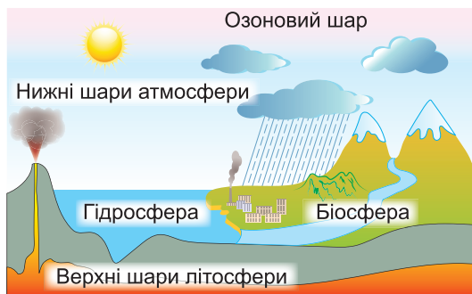
Мал. 12. Будова географічної оболонки
