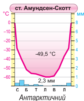
Мал. 27. Кліматодіаграми річного ходу температур і опадів у різних кліматичних поясах Землі
