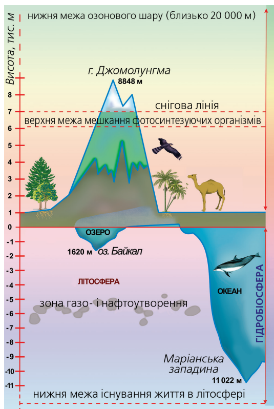
Мал. 41. Межі біосфери
