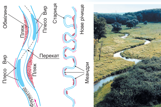
Мал. 19. Робота річки. Утворення меандр
