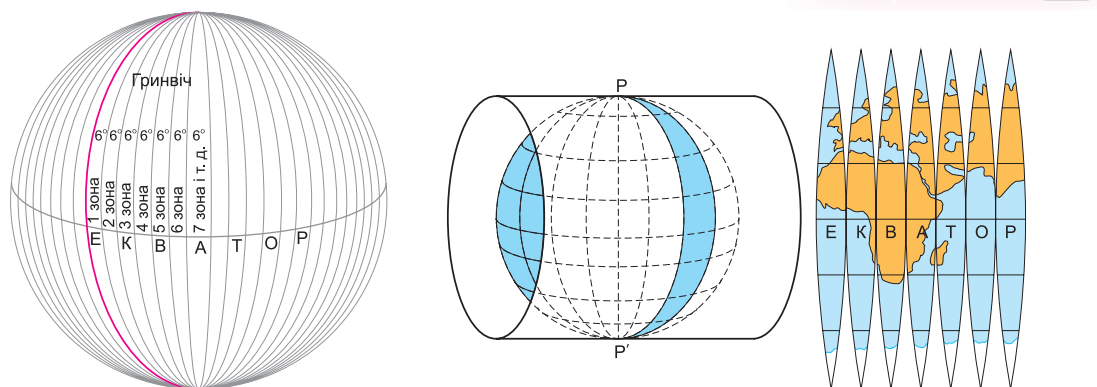
Мал. 2. Сутність проєкції Гаусса–Крюгера
