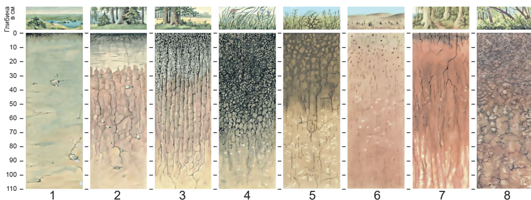
Мал. 45. Профілі різних ґрунтів Землі:
