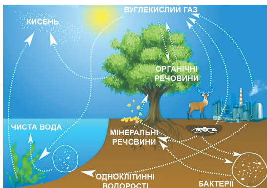
Мал. 14. Колообіг речовин у природі
