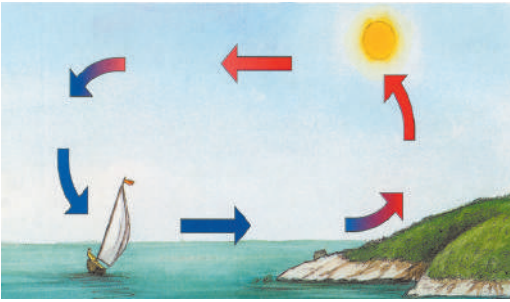
Рух повітря вдень
