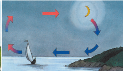
Рух повітря вночі
