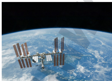
Міжнародна космічна станція на орбіті довкола Землі
