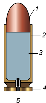
Будова унітарного патрона: 1 – куля; 2 – гільза; 3 – порох; 4 – фланець (закраїна); 5 – капсуль
