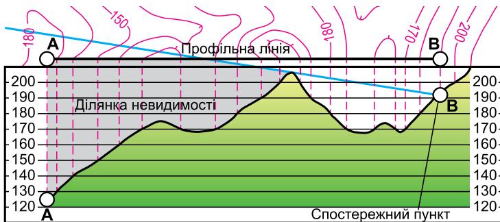
Побудова профілю місцевості
