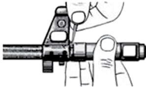
4. Відокремити дульне гальмо-компенсатор
