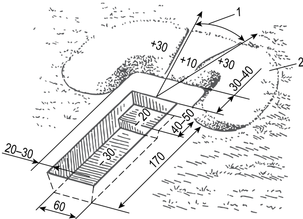
Одиночний окоп для стрільби з автомата лежачи: 1 – сектор обстрілу; 2 – бруствер (розміри в сантиметрах)
