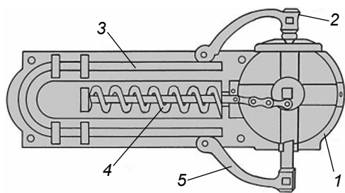
Коліщатковий замок Леонардо да Вінчі
