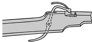
Гнотовий замок
