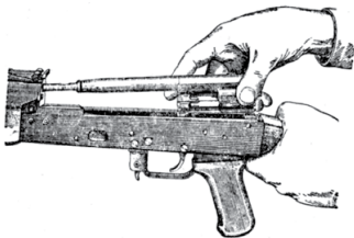
7. Відокремити затворну раму із затвором
