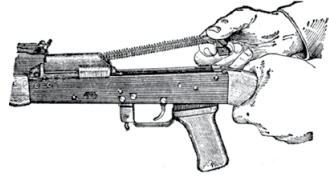
6. Відокремити зворотний механізм
