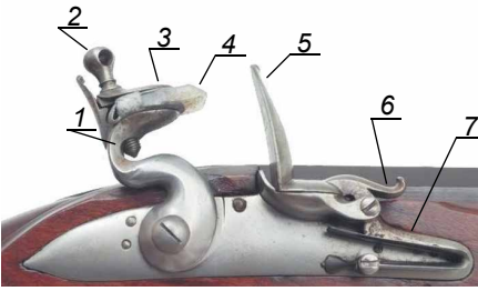
Кременевий замок: 1 – курок; 2 – курковий гвинт; 3 – верхня губа курка; 4 – кремін; 5 – кришка (кресало); 6 – полиця; 7 – підкресальна пружина
