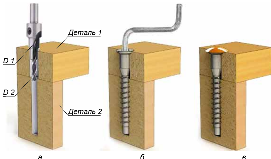
Мал. 63. З'єднання деталей єврогвинтом (конфірматом): а – свердління отвору; б – угвинчування; в – закриття заглушкою
