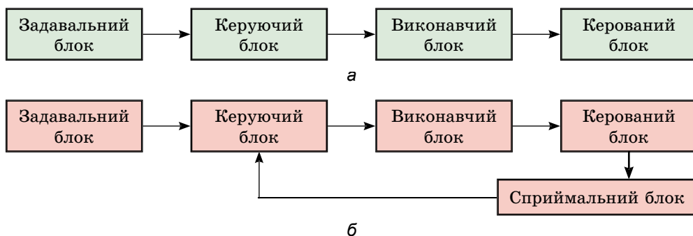
Мал. 87. Схеми автоматичної системи керування: а – з розімкнутим колом впливу; б – із замкнутим колом впливу
