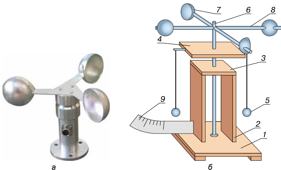
Мал. 70. Анеометр: а – загальний вигляд; б – будова: 1 – основа; 2 – стійка; 3 – поперечина; 4 – пластина; 5 – кулька; 6 – стрижень; 7 – лопать; 8 – хрестовина; 9 – шкала
