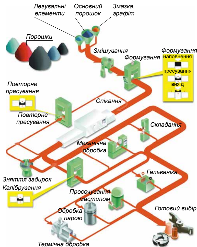
Мал. 3. Схема технологічного процесу виготовлення виробів методом порошкової металургії
